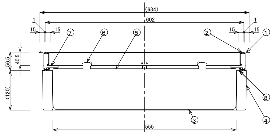
AA断面図
