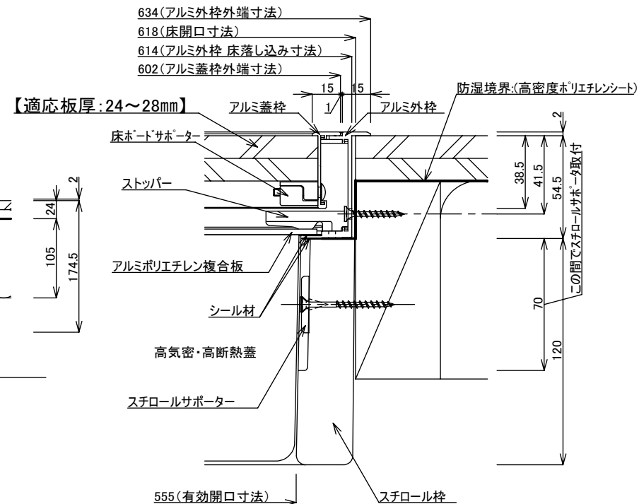
納まり詳細図(1/2)
