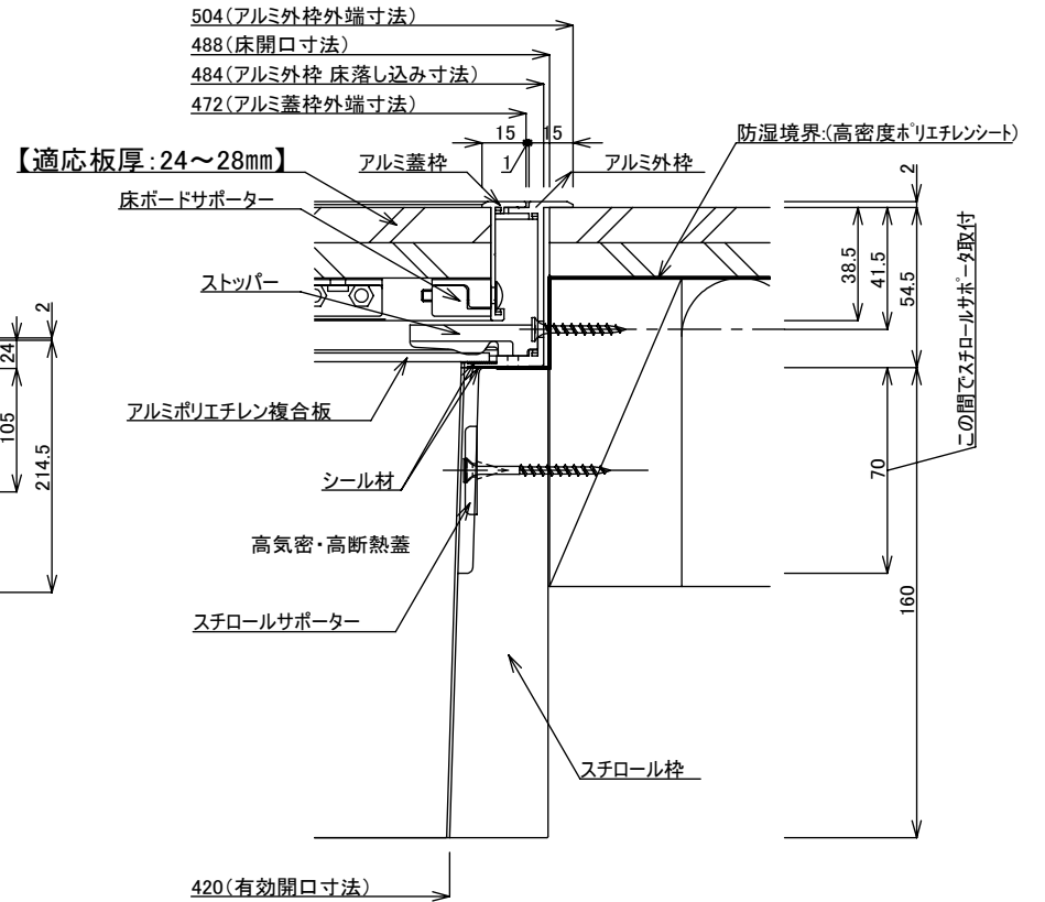
納まり詳細図(1/2)
